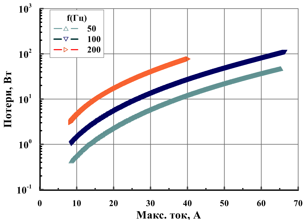
Рисунок 6.7 – Мощность измеренных потерь на синусоидальном токе в кольцевой статорной обмотке
