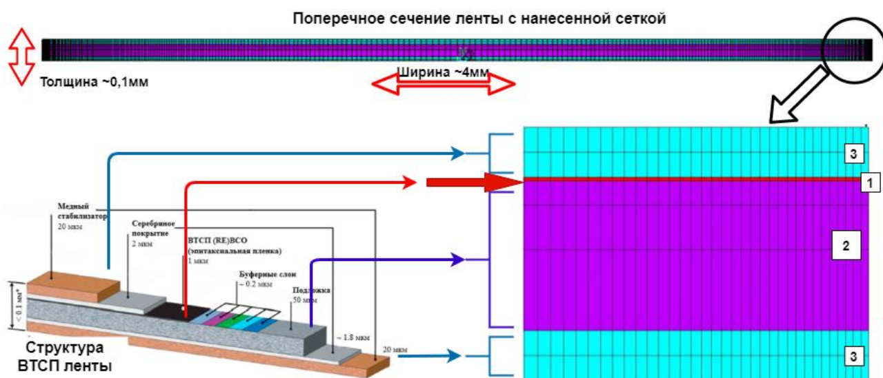
Рисунок 2.1 – Пример конечно-элементной сетки из МКЭ модели ВТСП ленты. На выделенном стрелкой укрупненном участке одной ленты «1» – ВТСП слой, «2» – подложка, «3» – стабилизирующие слои
