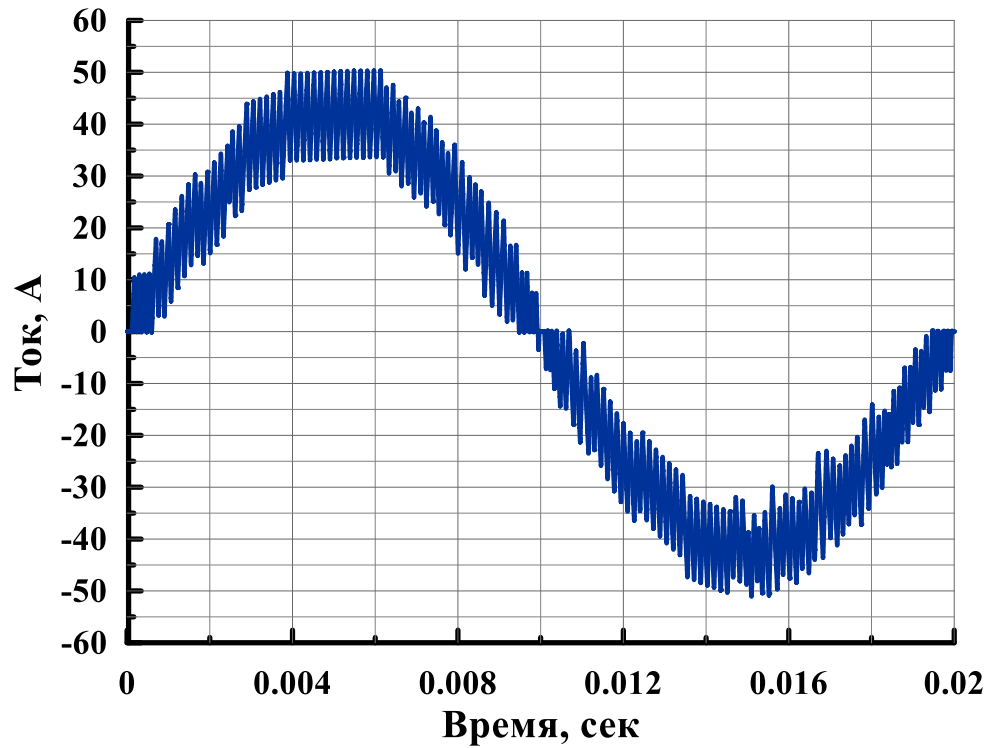
Рисунок 5.11 – Сформированный в ВТСП катушке синусоидальный ток с частотой 50 Гц (режим «СМ»)
