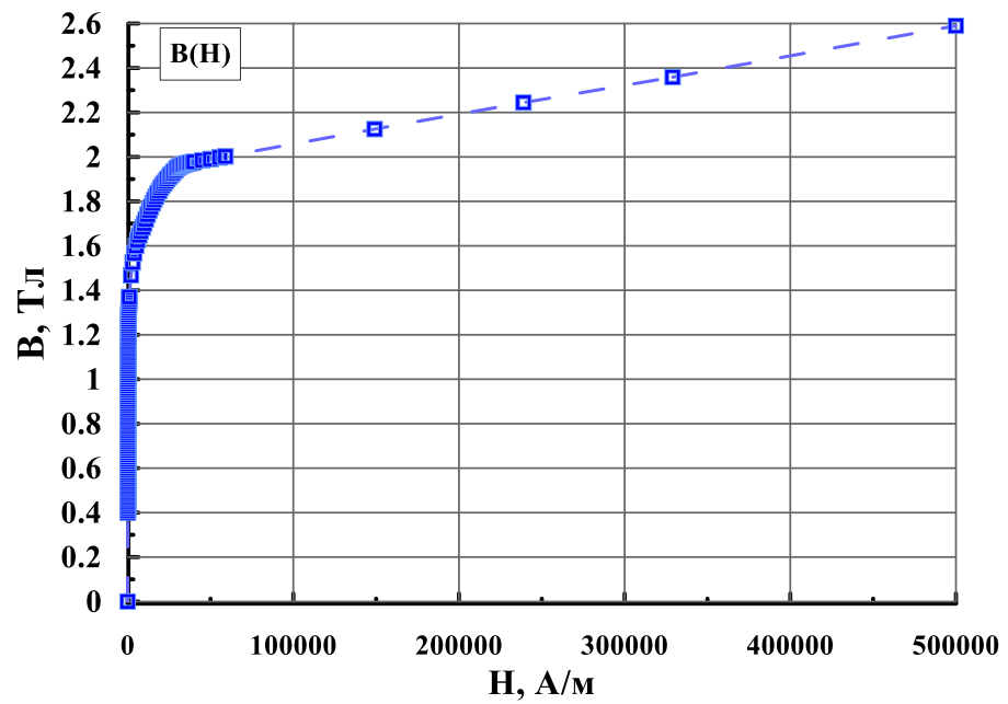
Рисунок 6.9 – Кривая намагниченности стали 2412
