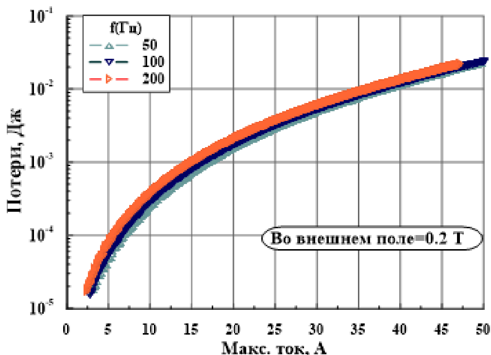
Рисунок 6.11 – Измеренные потери в одной катушке, используемой в кольцевой статорной обмотке во внешнем поле 0,2 Тл
