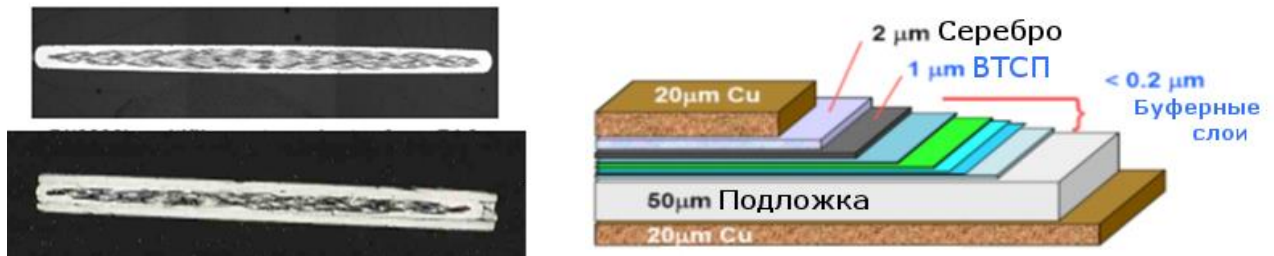
Рисунок 1.13 – Поперечное сечение 1G (слева) и 2G (справа) ВТСП лент
