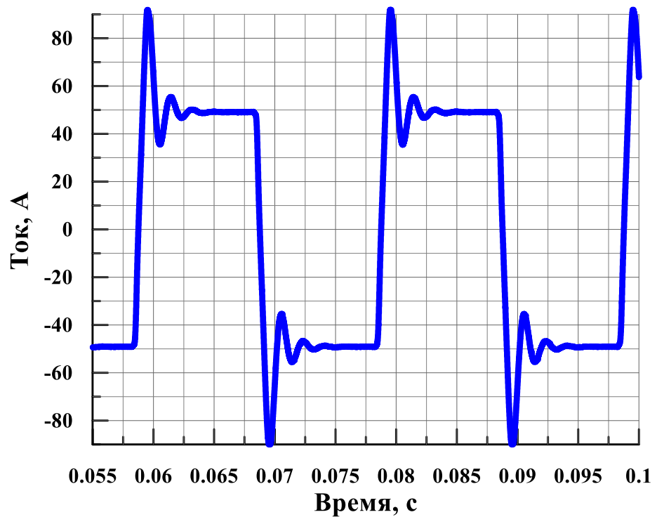
Рисунок 4.9 – Форма тока в катушке при частоте 50 Гц
