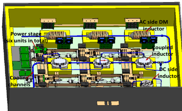
Рисунок 1.10 – Топология (слева) преобразователя с криогенным охлаждением и его компоновка (справа)
