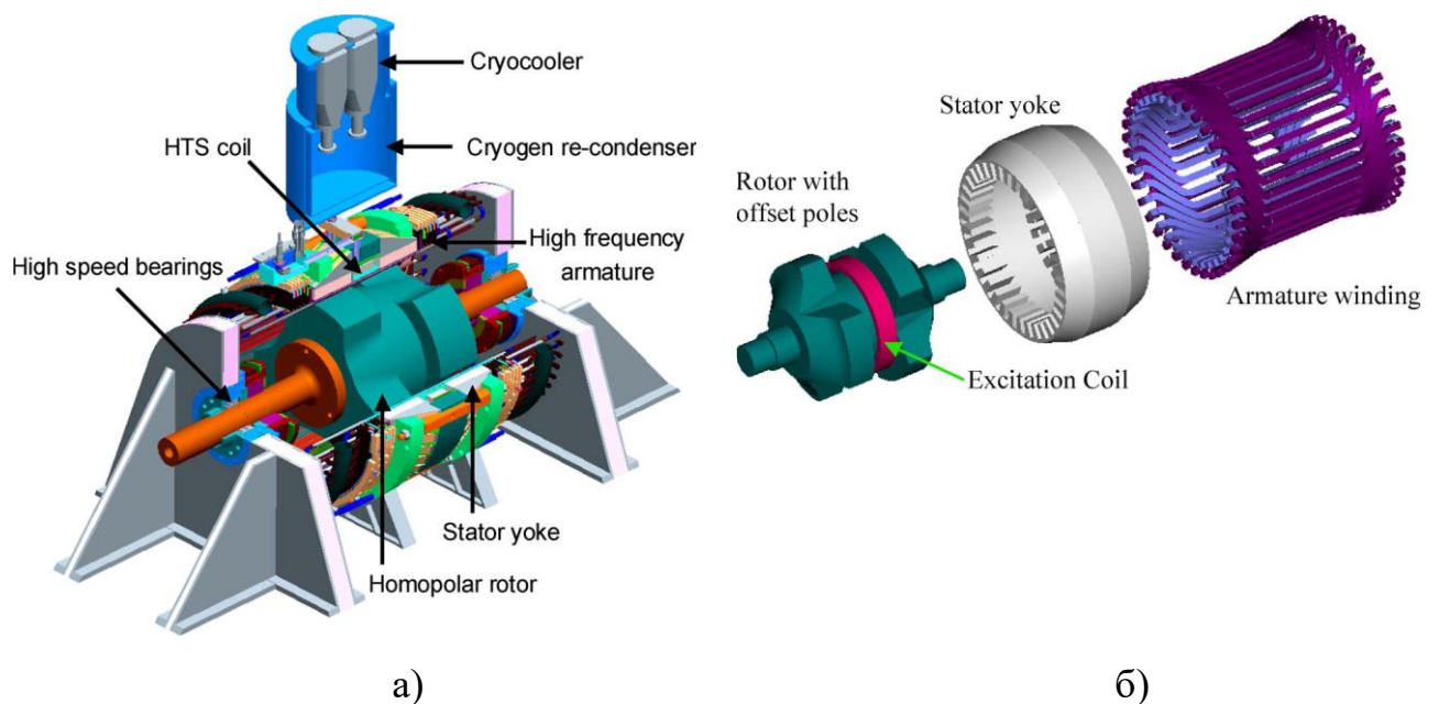
Рисунок 1.5 – Униполярный генератор авиационного назначения от компании General Electric: а) общий вид, б) конструкция активной зоны
