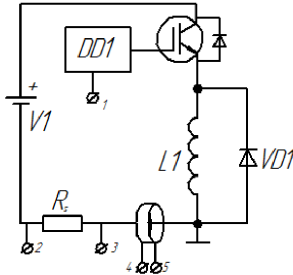
Рисунок 5.4 – Схема испытательного стенда для датчиков тока
