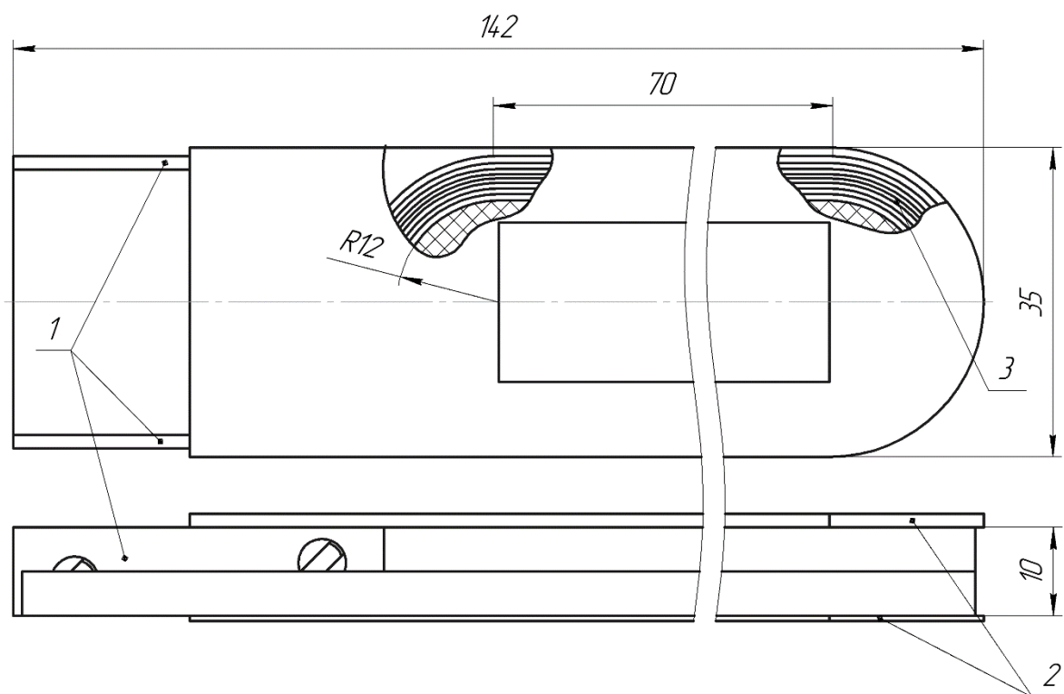
Рисунок 4.4 – Эскиз ВТСП катушки, изготовленной с использованием разработанного намоточного станка: 1 – медные клеммы, 2 – каркас катушки, 3 – ВТСП лента
