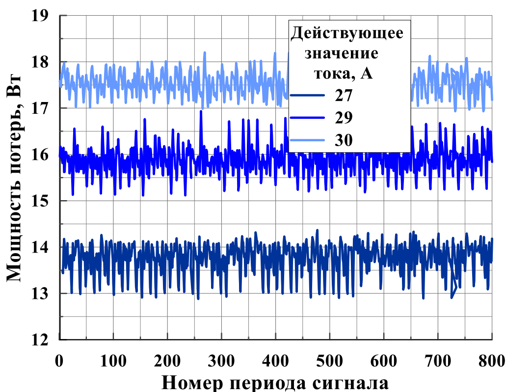
Рисунок 5.14 – Потери в ВТСП катушке по периодам для трех значений трапецеидального тока при частоте 200 Гц
