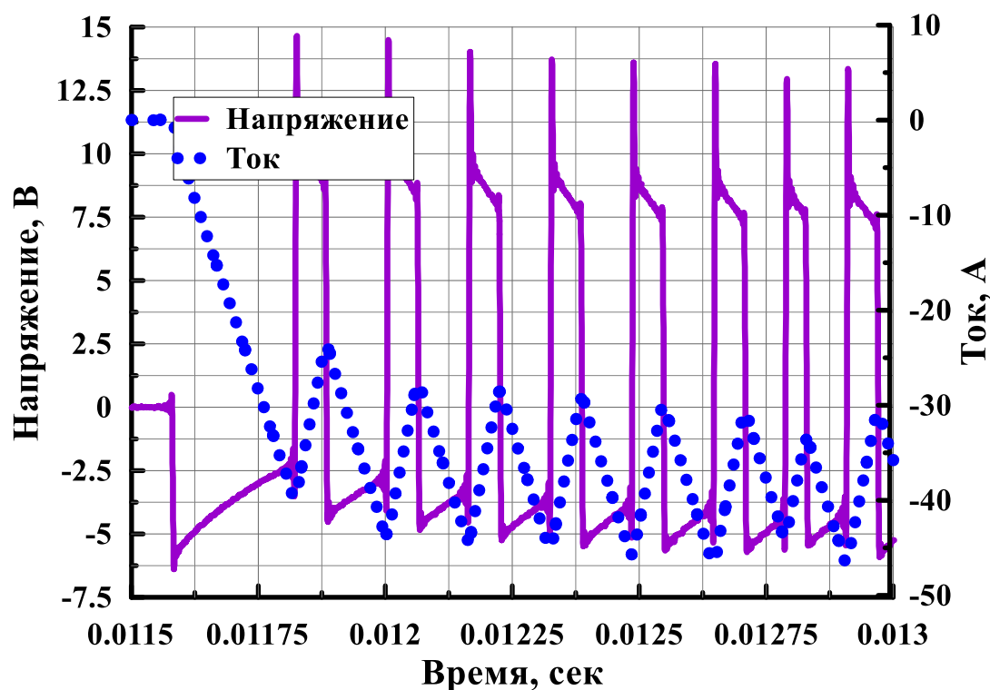
Рисунок 5.13 – Напряжение и ток в ВТСП катушке
