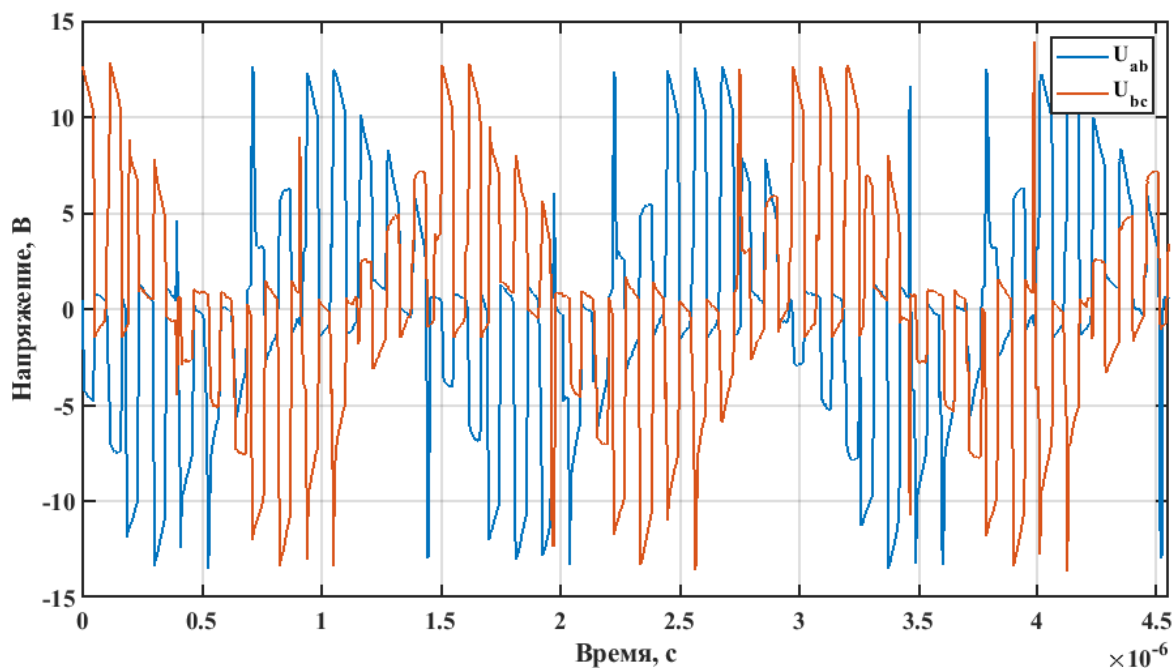
Рисунок 1.11 – Осциллограммы фазных напряжений на выходе 300 Вт инвертора для авиамоделей. Напряжение на третьей фазе не показано для наглядности
