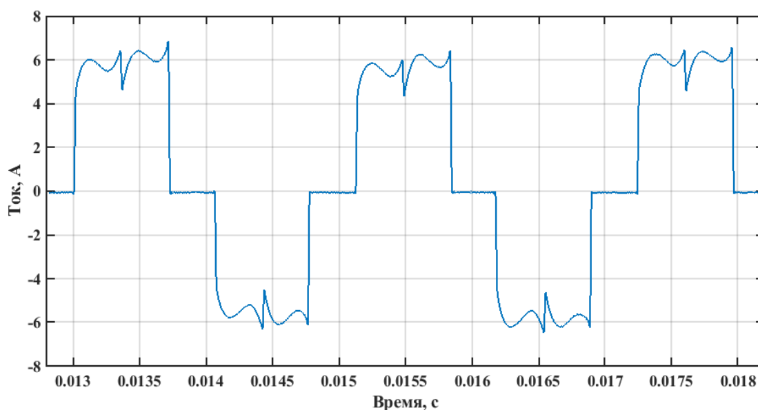
Рисунок 1.12 – Ток фазы бесколлекторного двигателя постоянного тока
