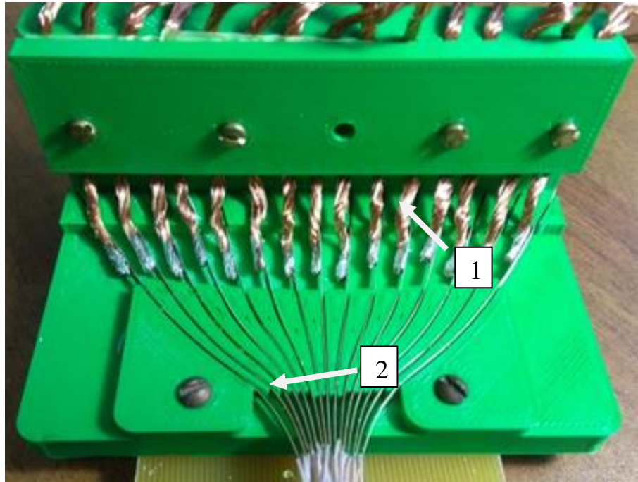
Рисунок 2.3 – Фотография собранного токоввода: 1 – концы лент с индивидуальными медными токовводами; 2 – зона припайки потенциальных контактов
