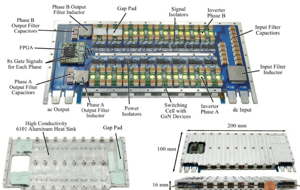
Рисунок 1.9 – Инвертор мощностью 10 кВт
