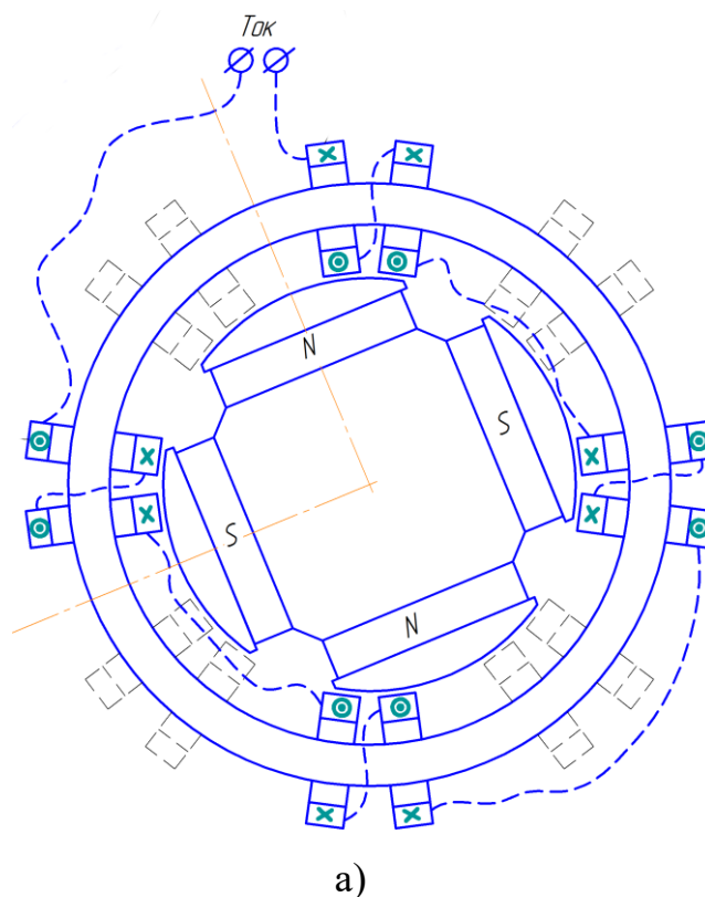
Рисунок 6.6. а) Схематичное изображение статорной обмотки с установленным внутри ротором; сплошными линиями обозначена обмотка одной из двух фаз. б) Собранный пакет кольцевой статорной обмотки
