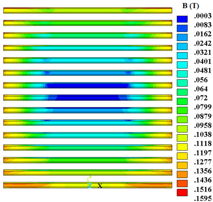
Рисунок 3.4 – Распределение магнитного поля в стопке из 15 ВТСII лент для момента времени, когда амплитуда тока составляет 80А
