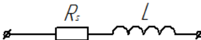
Рисунок 5.2 – Эквивалентная схема шунтового датчика на переменном токе
