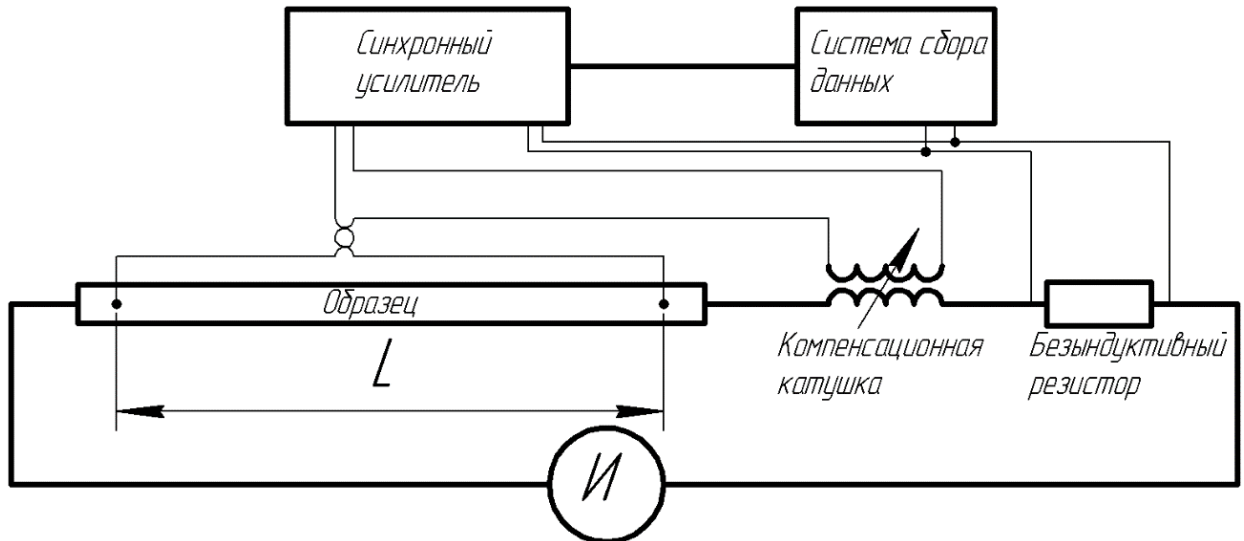
Рисунок 1.19 - Измерение потерь образца в собственном поле с использованием синхронного усилителя
