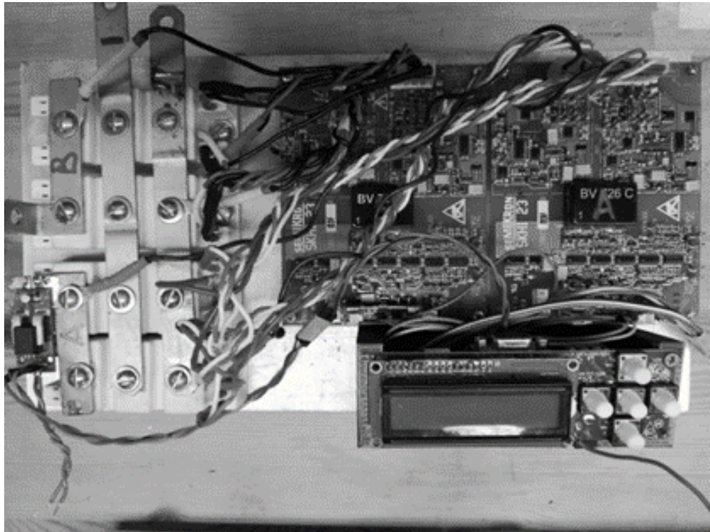
Рисунок 5.10 – Общий вид инвертора
